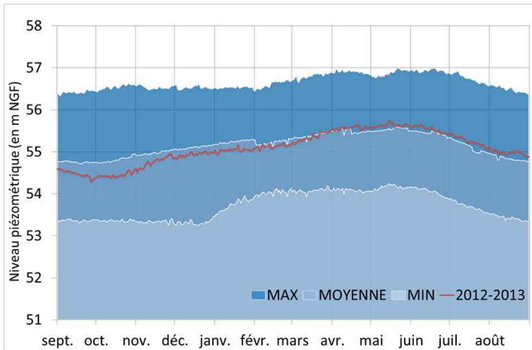
Graphique 38 - Piézomètre Ponteilla : suivi piézométrique de l'année 2012-2013
