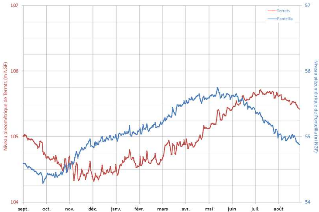
Graphique 52 – Secteur des Aspres : fluctuation piézométrique année 2012-2013
