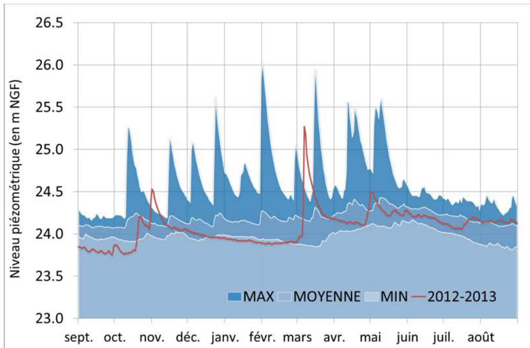
Graphique 9 - Piézomètre Ortaffa : historique de l'évolution piézométrique
