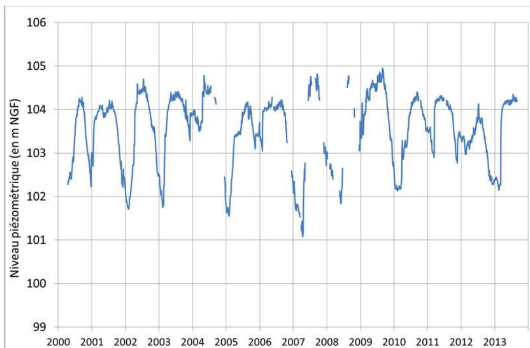
Graphique 11 - Piézomètre Millas C2-1 : historique de l'évolution piézométrique
