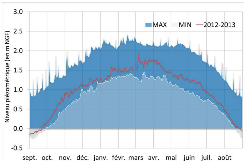
Graphique 14 - Piézomètre Barcarès PN4 : suivi piézométrique de l'année 2012-2013
