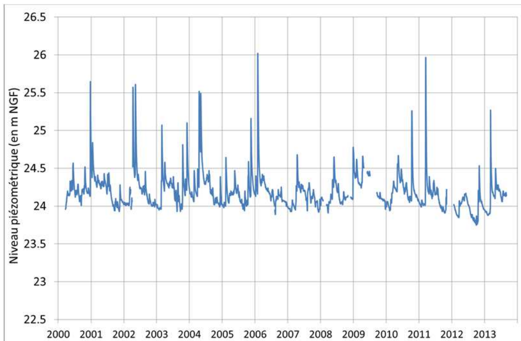
Graphique 9 - Piézomètre Ortaffa : historique de l'évolution piézométrique
