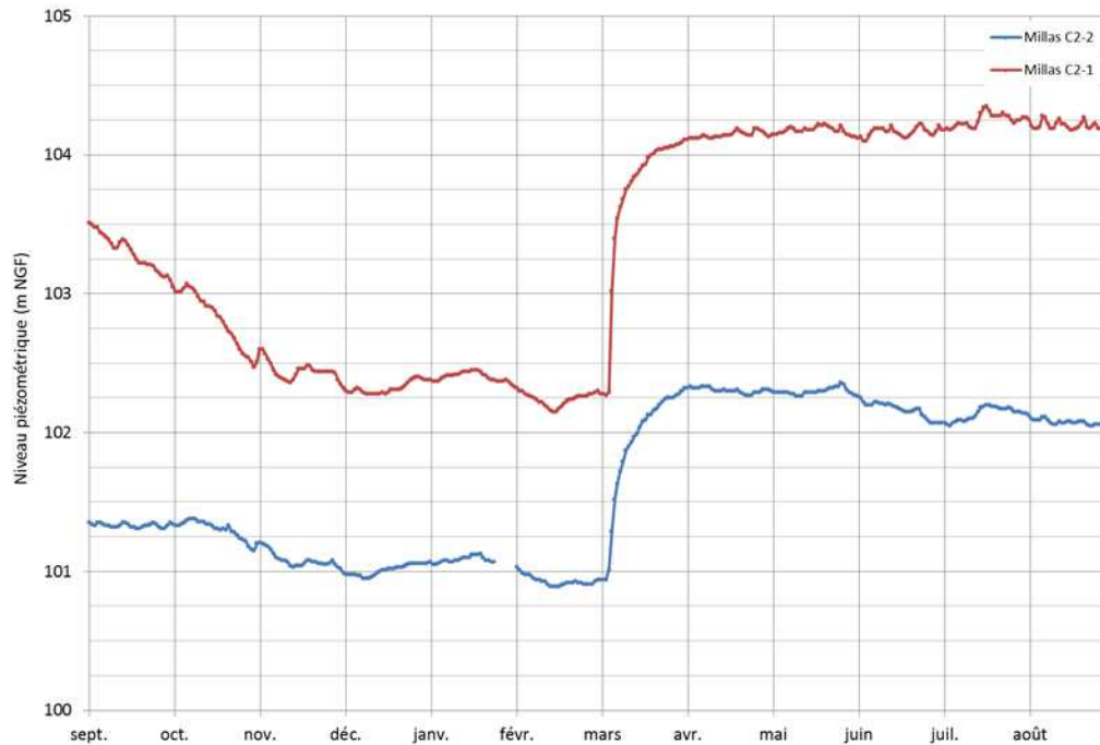
Graphique 50 – Secteur du BV amont de la Têt : fluctuation piézométrique année 2012-2013
