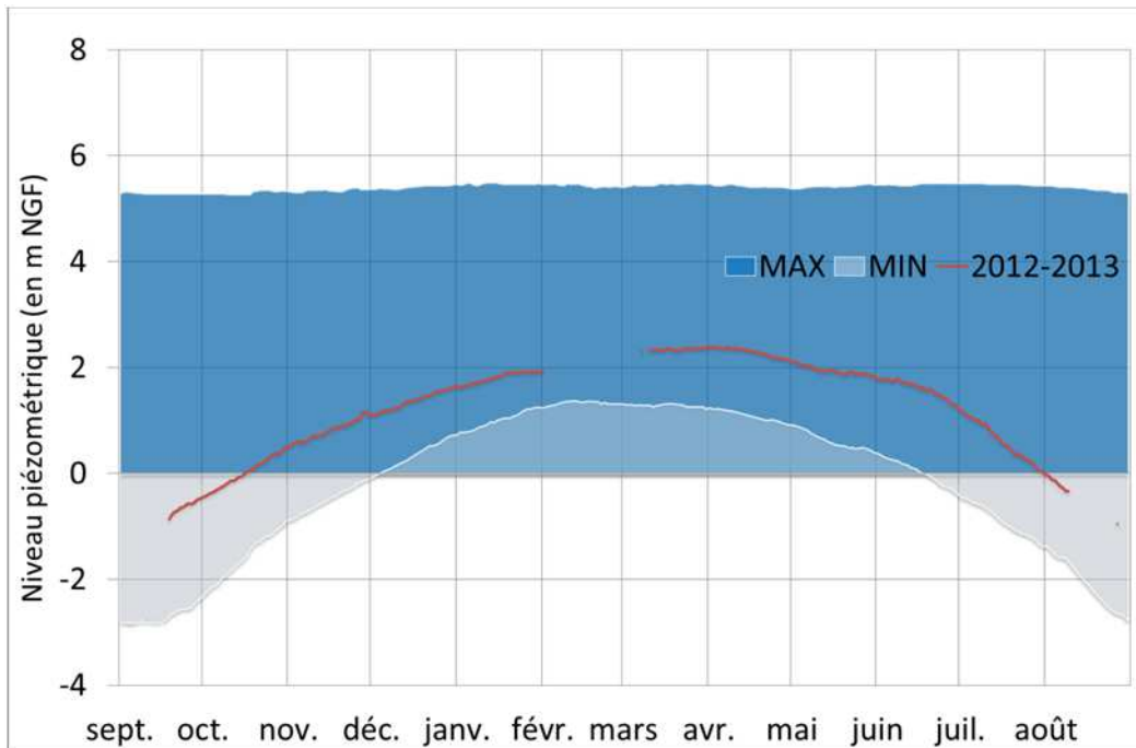
Graphique 33 - Piézomètre Saint Laurent : historique de l'évolution piézométrique
