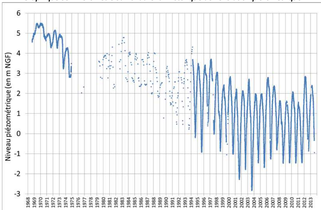
Graphique 33 - Piézomètre Saint Laurent : historique de l'évolution piézométrique
