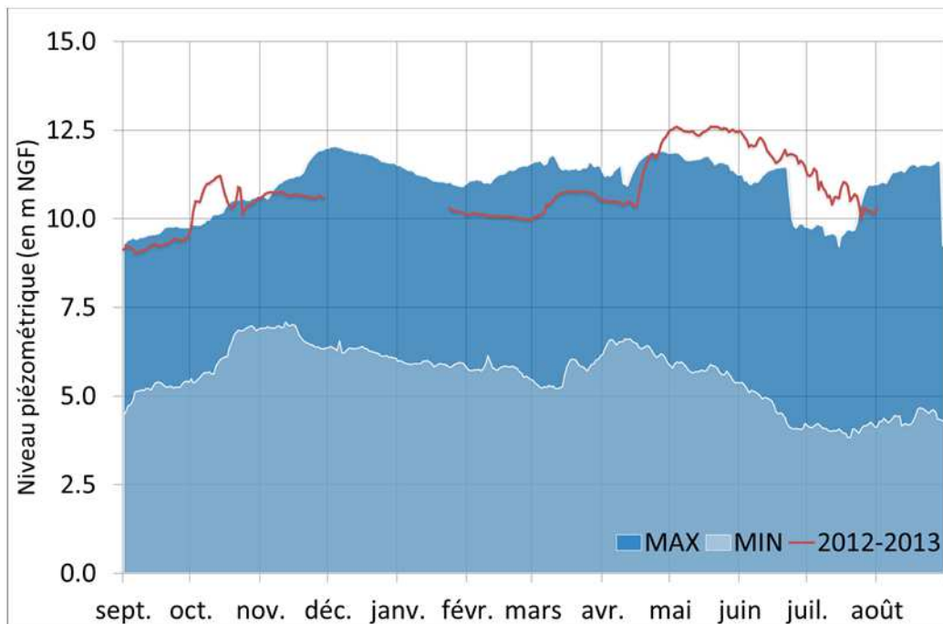
Graphique 46 - Piézomètre Pia : suivi piézométrique de l'année 2012-2013
