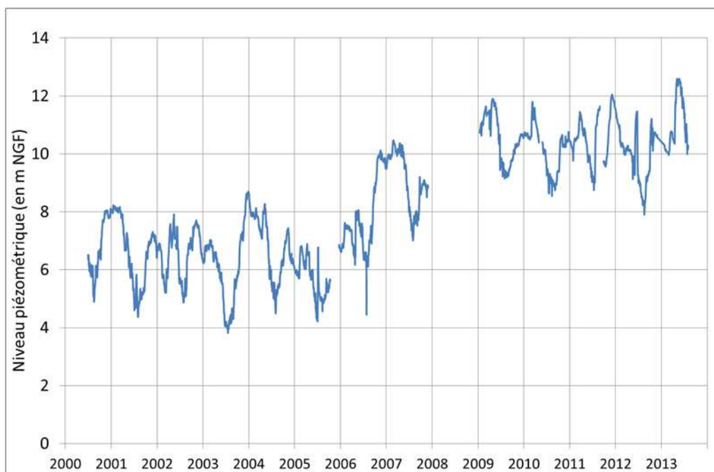
Graphique 47 - Piézomètre Pia : historique de l'évolution piézométrique
