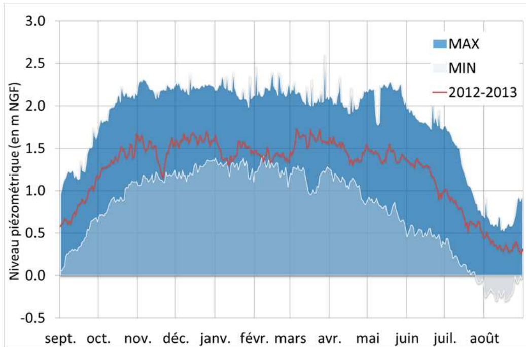
Graphique 20 - Piézomètre Canet : suivi piézométrique de l'année 2012-2013
