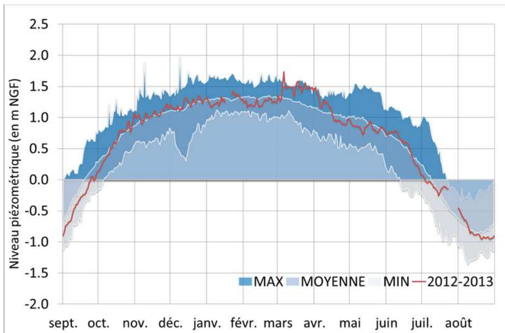
Graphique 12 - Piézomètre Barcarès PN3 : suivi piézométrique de l'année 2012-2013
