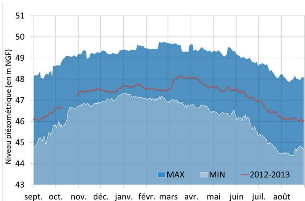
Graphique 36 - Piézomètre Perpignan : suivi piézométrique de l'année 2012-2013
