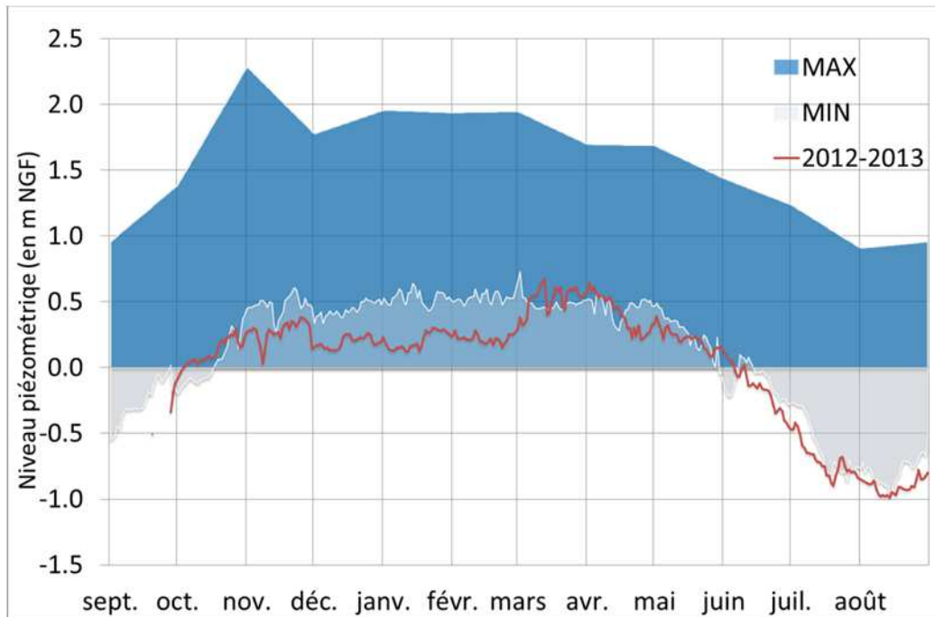
Graphique 23 – Sainte Marie N4 : historique de l'évolution piézométrique
