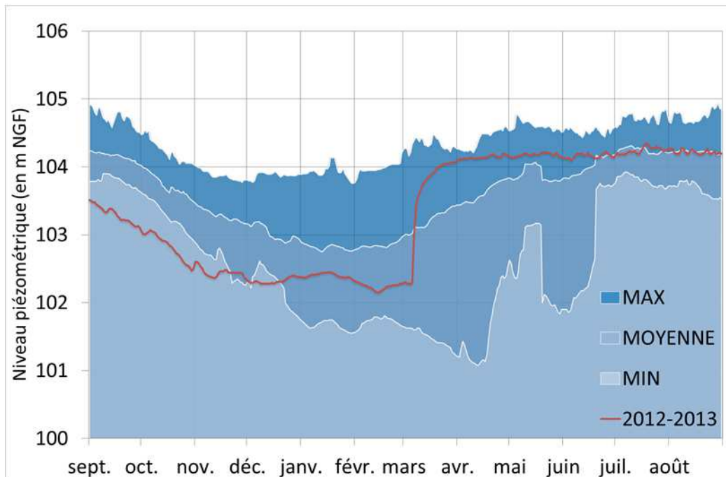
Graphique 10 - Piézomètre Millas C2-1 : suivi piézométrique de l'année 2012-2013
