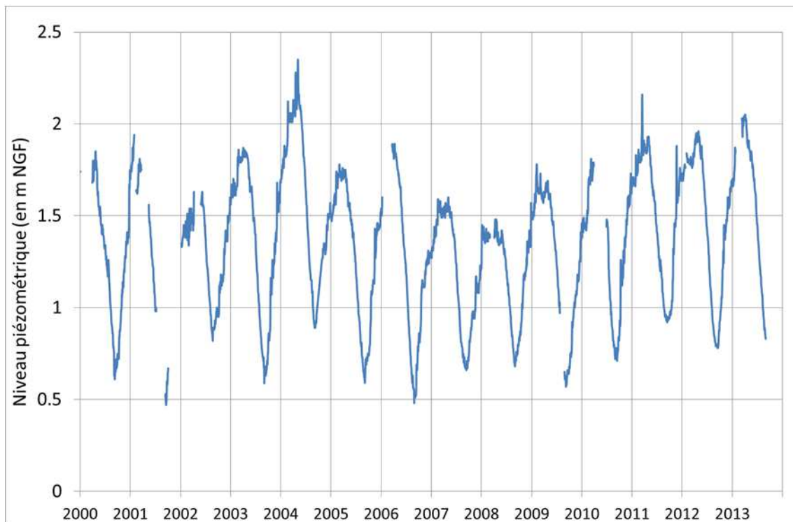
Graphique 25 - Piézomètre Saint Nazaire : historique de l'évolution piézométrique
