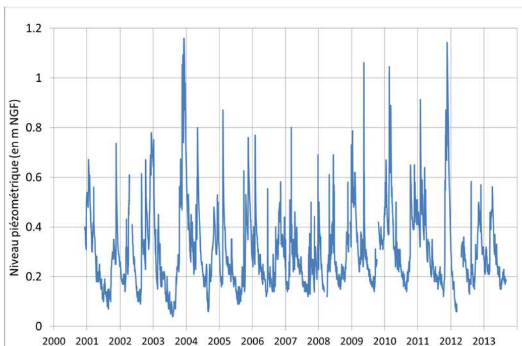
Graphique 7 - Piézomètre Barqua : historique de l'évolution piézométrique
