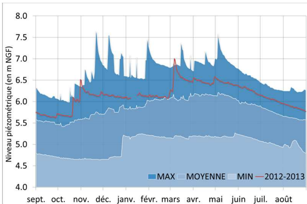
Graphique 2 – Piézomètre d'Alénia : suivi piézométrique de l'année 2012-2013
