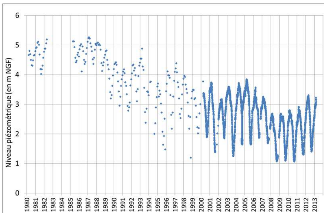
Graphique 17 - Piézomètre Barcarès SN4 : historique de l'évolution piézométrique
