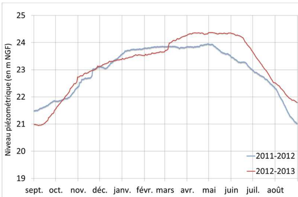
Graphique 26 - Piézomètre Sabirou : suivi piézométrique de l'année 2012-2013
