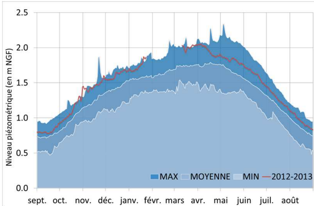
Graphique 24 - Piézomètre Saint Nazaire : suivi piézométrique de l'année 2012-2013
