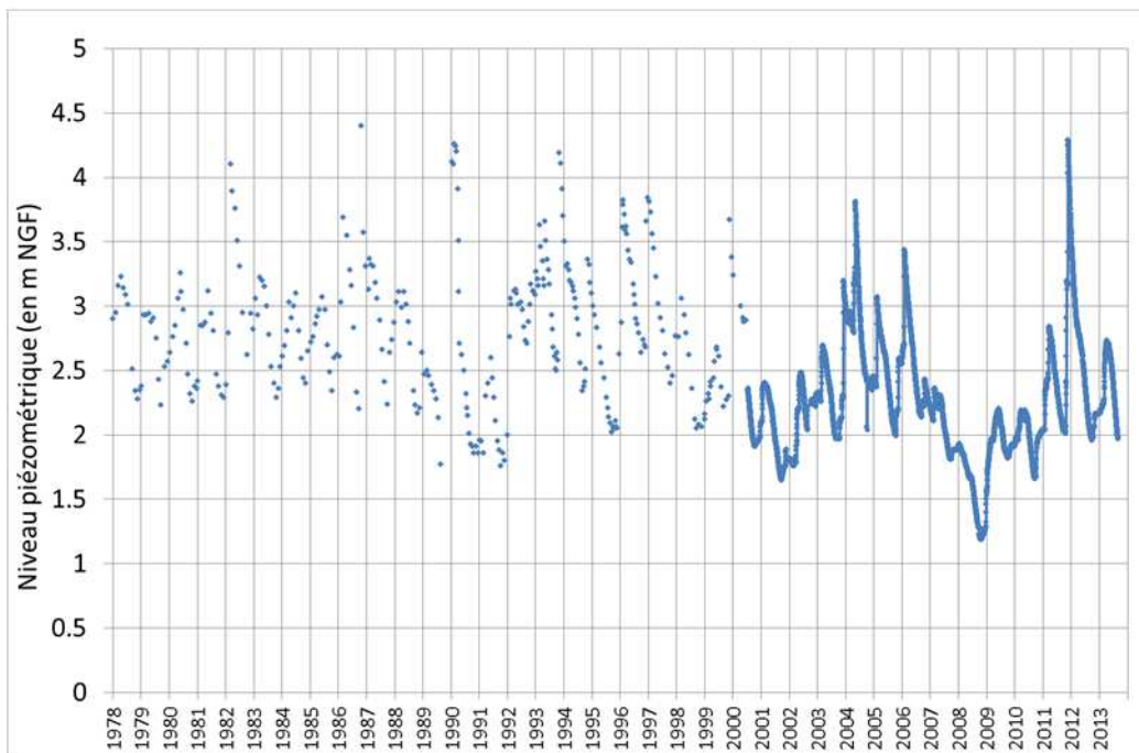
Graphique 5 - Piézomètre de Saint Hippolyte : historique de l'évolution piézométrique
