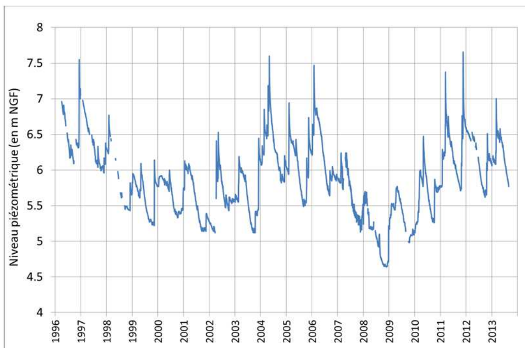
Graphique 3 – Piézomètre d'Alénia : historique de l'évolution piézométrique
