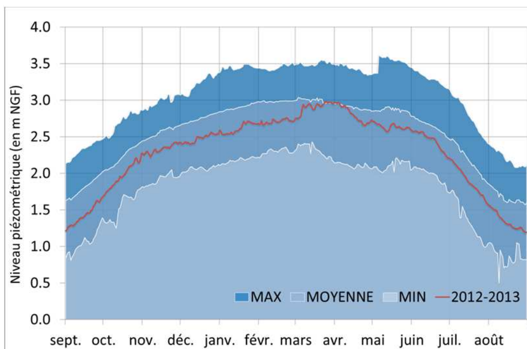
Graphique 40 - Piézomètre Torreilles : suivi piézométrique de l'année 2012-2013
