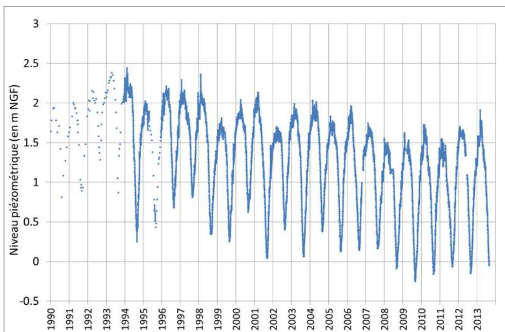
Graphique 15 - Piézomètre Barcarès PN4 : historique de l'évolution piézométrique
