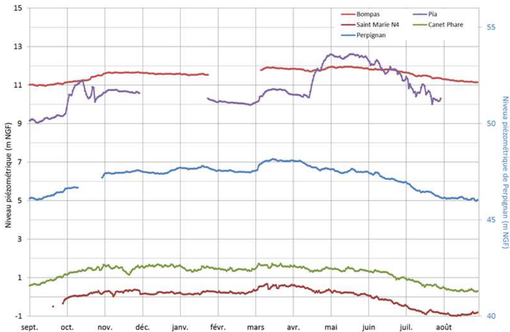
Graphique 49 – Secteur du BV aval de la Têt : fluctuation piézométrique année 2012-2013
