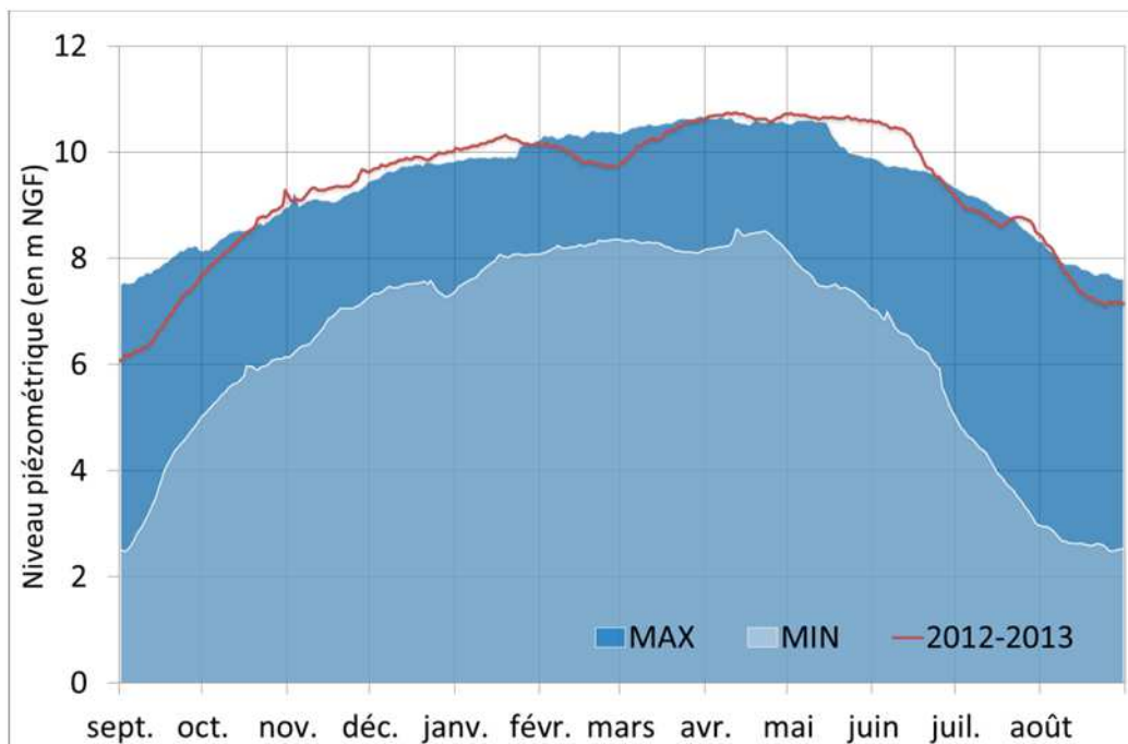
Graphique 44 - Piézomètre Corneilla : suivi piézométrique de l'année 2012-2013
