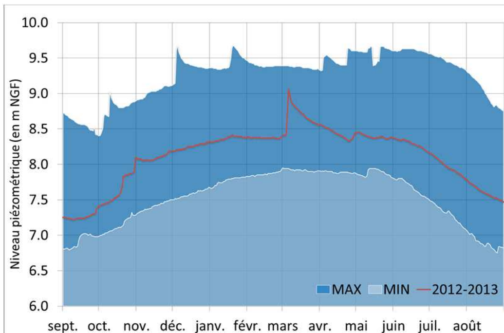
Graphique 28 - Piézomètre Argelès sur Mer : suivi piézométrique de l'année 2012-2013
