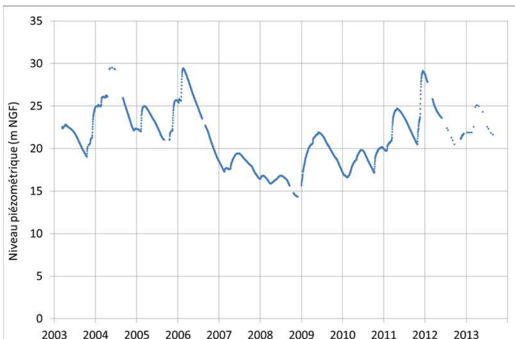
Graphique 31 - Piézomètre Ex-Opoul : historique de l'évolution piézométrique
