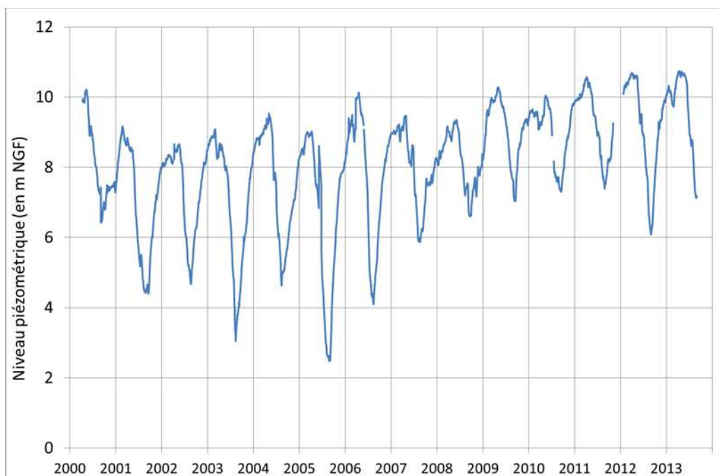
Graphique 45 - Piézomètre Corneilla : historique de l'évolution piézométrique
