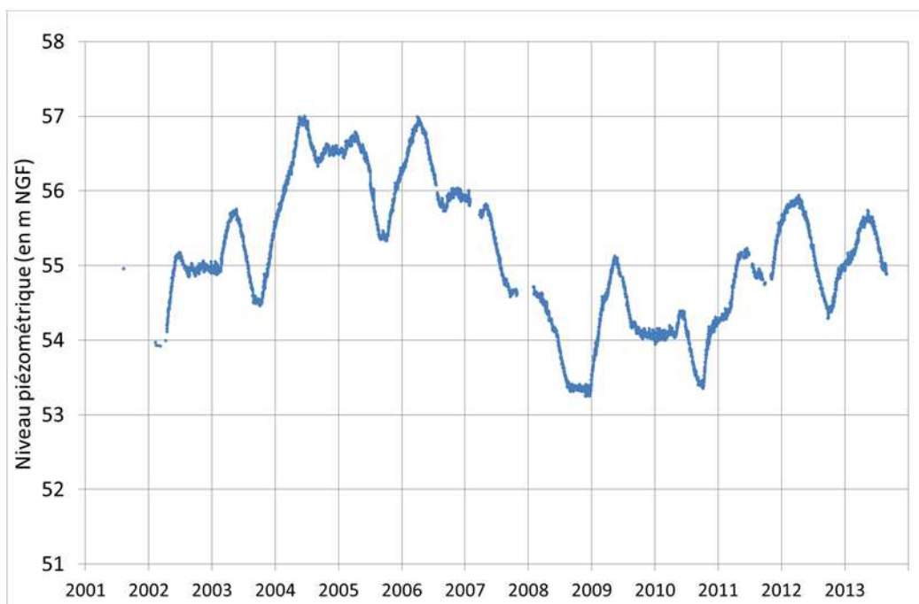
Graphique 39 - Piézomètre de Ponteilla : historique de l'évolution piézométrique
