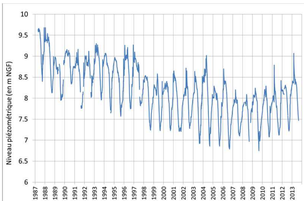
Graphique 29 - Piézomètre d'Argelès sur Mer : historique de l'évolution piézométrique
