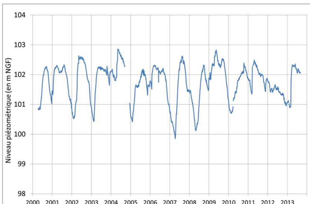
Graphique 35 - Piézomètre Millas C2-2 : historique de l'évolution piézométrique
