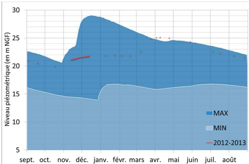
Graphique 30 - Piézomètre Ex-Opoul : suivi piézométrique de l'année 2012-2013
