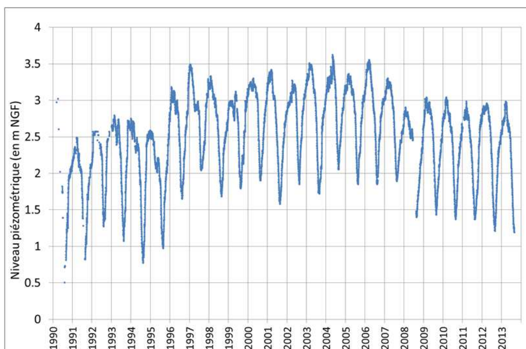
Graphique 41 - Piézomètre Torreilles : historique de l'évolution piézométrique
