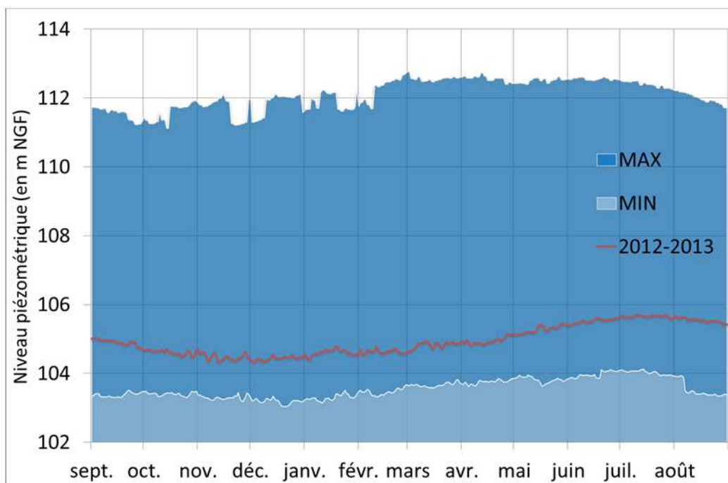
Graphique 42 - Piézomètre Terrats : suivi piézométrique de l'année 2012-2013
