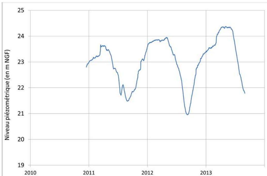
Graphique 27 - Piézomètre Sabirou : historique de l'évolution piézométrique
