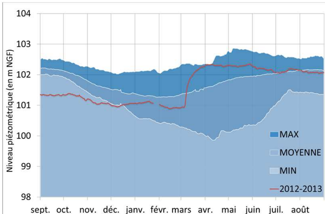
Graphique 34 - Piézomètre Millas C2-2 : suivi piézométrique de l'année 2012-2013
