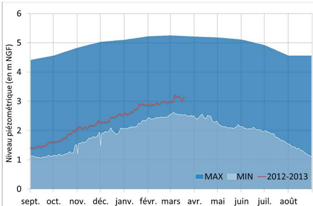
Graphique 16 - Piézomètre Barcarès SN4 : suivi piézométrique de l'année 2012-2013
