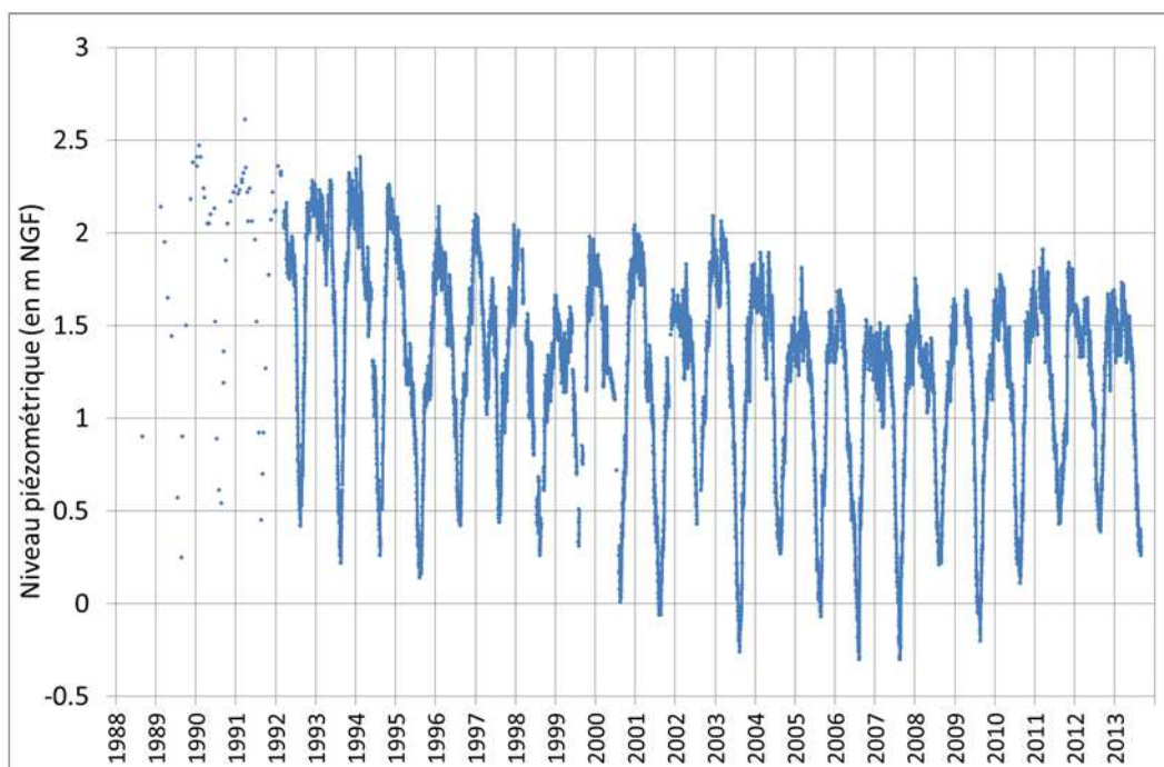
Graphique 21 - Piézomètre Canet : historique de l'évolution piézométrique
