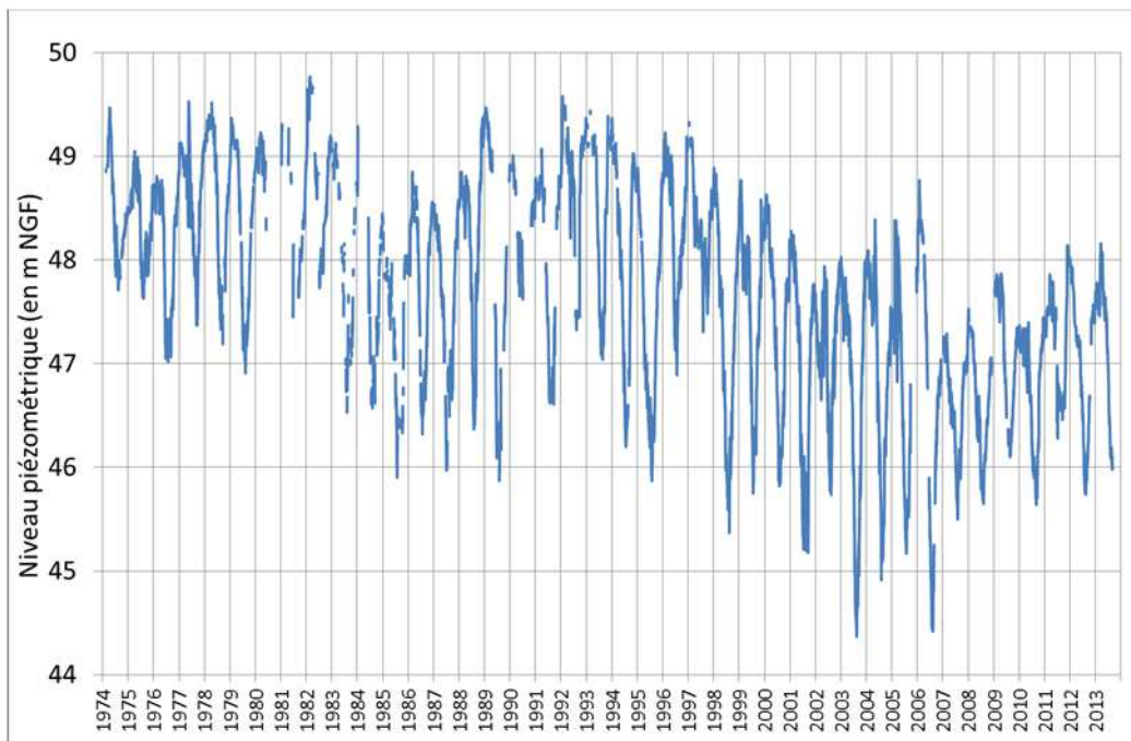
Graphique 37 - Piézomètre Perpignan : historique de l'évolution piézométrique
