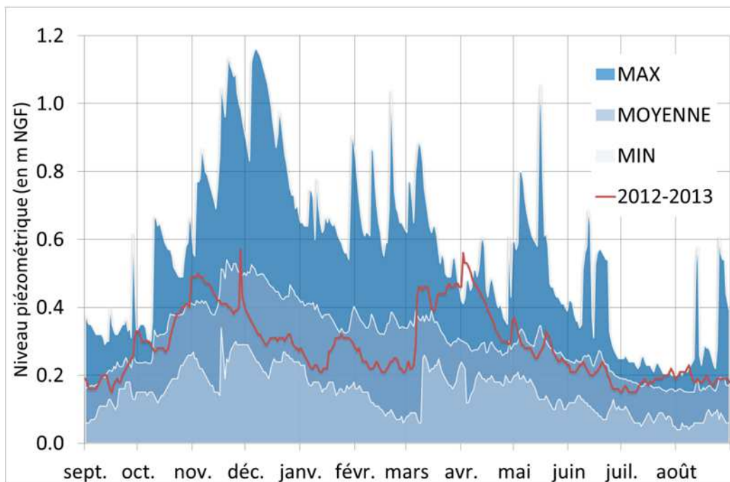
Graphique 6 - Piézomètre Barqua : suivi piézométrique de l'année 2012-2013
