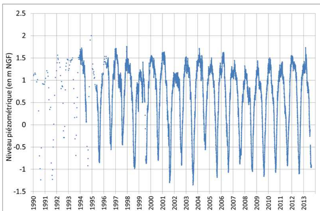
Graphique 13 - Piézomètre Barcarès PN3 : historique de l'évolution piézométrique
