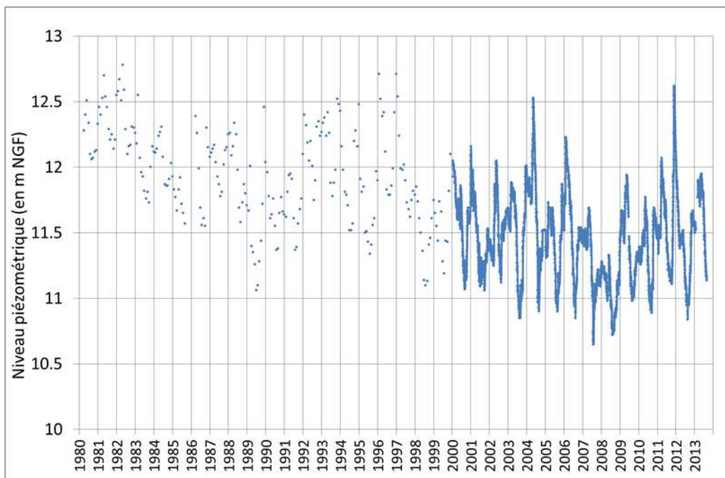
Graphique 19 - Piézomètre Bompas : historique de l'évolution piézométrique
