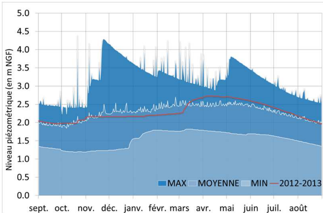
Graphique 4 - Piézomètre Saint Hippolyte : suivi piézométrique de l'année 2012-2013
