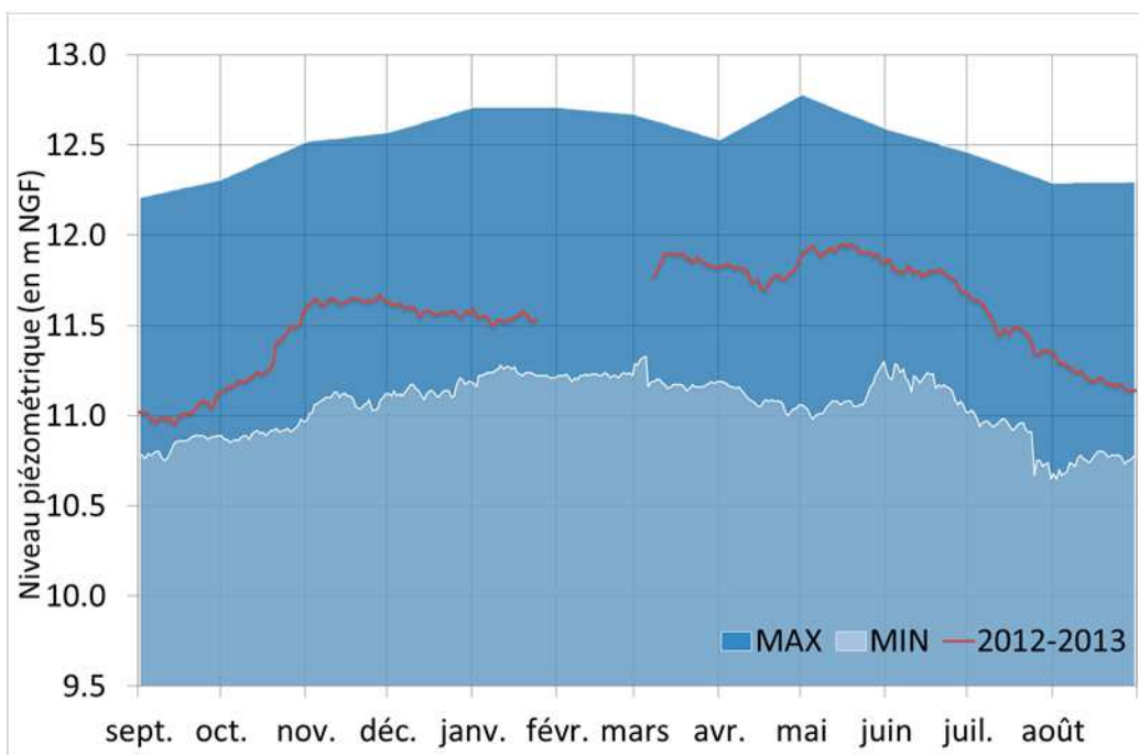
Graphique 18 - Piézomètre Bompas : suivi piézométrique de l'année 2012-2013
