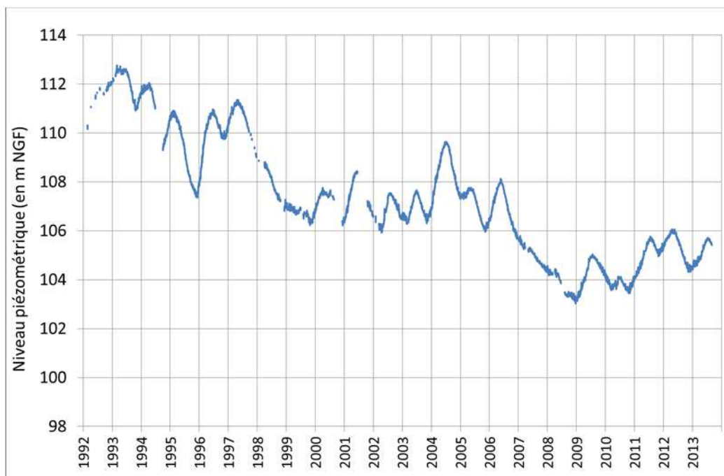
Graphique 43 - Piézomètre Terrats : historique de l'évolution piézométrique
