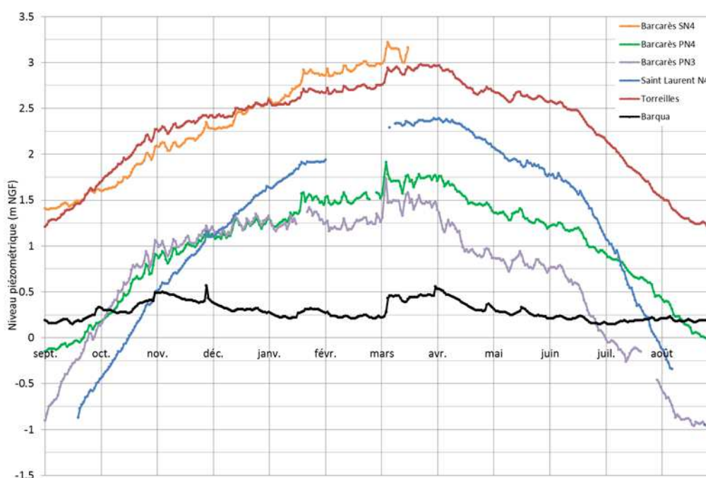
Graphique 48 – Secteur littoral Salanque : fluctuation piézométrique année 2012-2013
